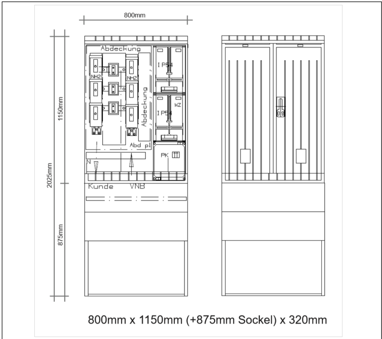
Zeichnung
