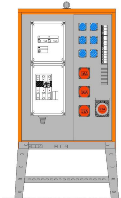
BSV-VS-0011 Verteilerschrank Baustromstand
