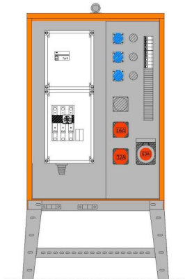
BSV-VS-0008 Verteilerschrank Baustromstand
