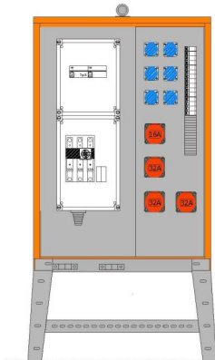
BSV-VS-0006 Verteilerschrank Baustromstandve
