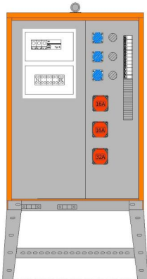
BSV-VS-0002 Verteilerschrank Baustromstandve
