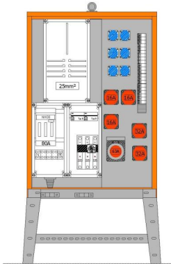
BSV-AV-0011 Anschlussverteilerschrank Baustro
