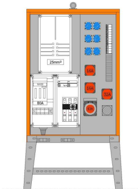
BSV-AV-0008 Anschlussverteilerschrank Baustr
