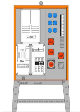
BSV-AV-0007 Anschlussverteilerschrank Baustro
