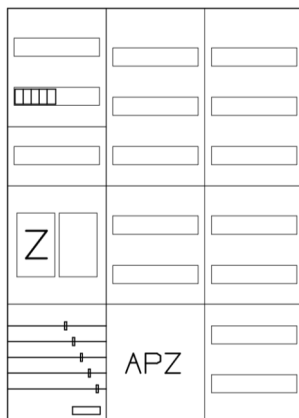
AEZ32-210-015, eHZ-Verteilung HEART
