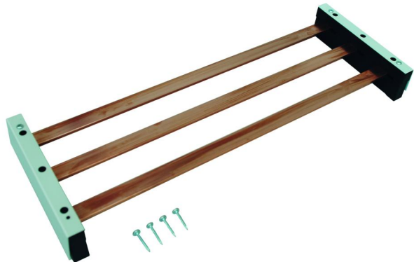
Sammelschiene CU 3-polig, BxH=30x5mm, 1-Feld
