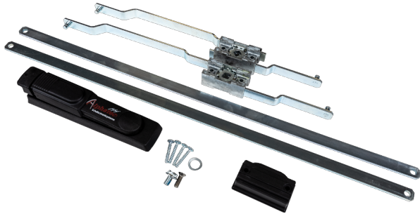
Schwenkhebel für PHZ, mit St. u. Flachstangensatz
